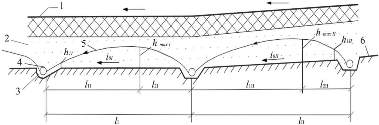
Рисунок 2 – Формування міграції води в дренажному шарі на ділянці з поздовжнім похилом більшим за поперечний: 1 – покриття; 2 – основа; 3 – дренажна траншея; 4 – дренажна труба; 5 – крива депресії; 6 – земляне полотно
